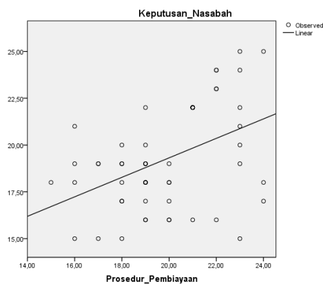
Gambar 5.8: Kurva linieritas Variabel Y atas Variabel X
