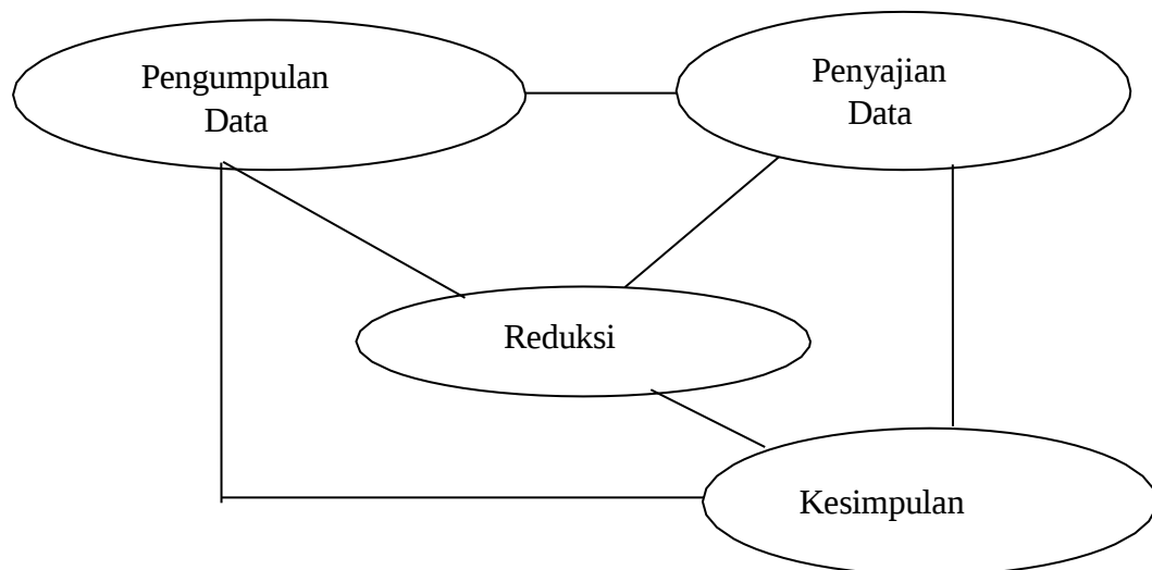
Gambar 3.1 komponen dalam analisis data (model interaktif) (Sugiyono, 2015 : 338)
